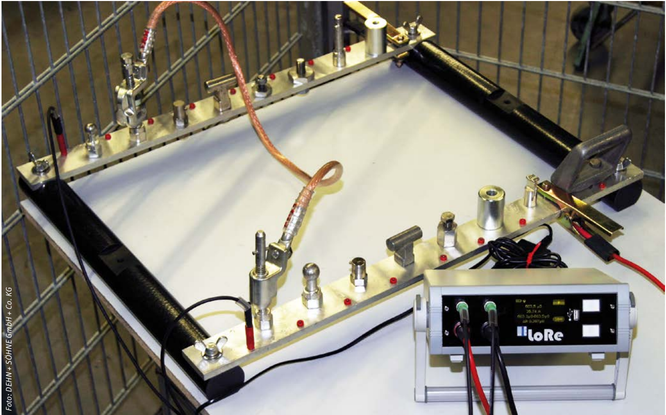
Abbildung 1: Prüfaufbau
